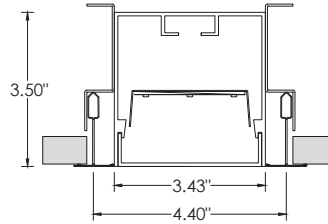
15L - 15/16" LAYIN
