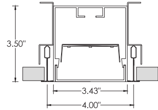
9L - 9/16" LAYIN
